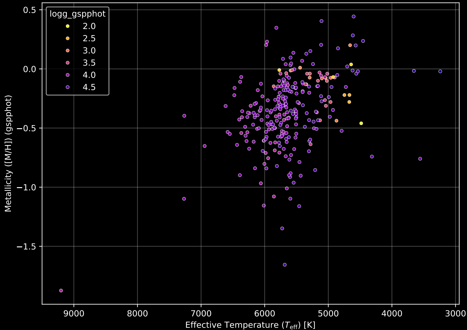
GALAH DR4 Field: [142] Stellar Population Parameters (n= 272)
