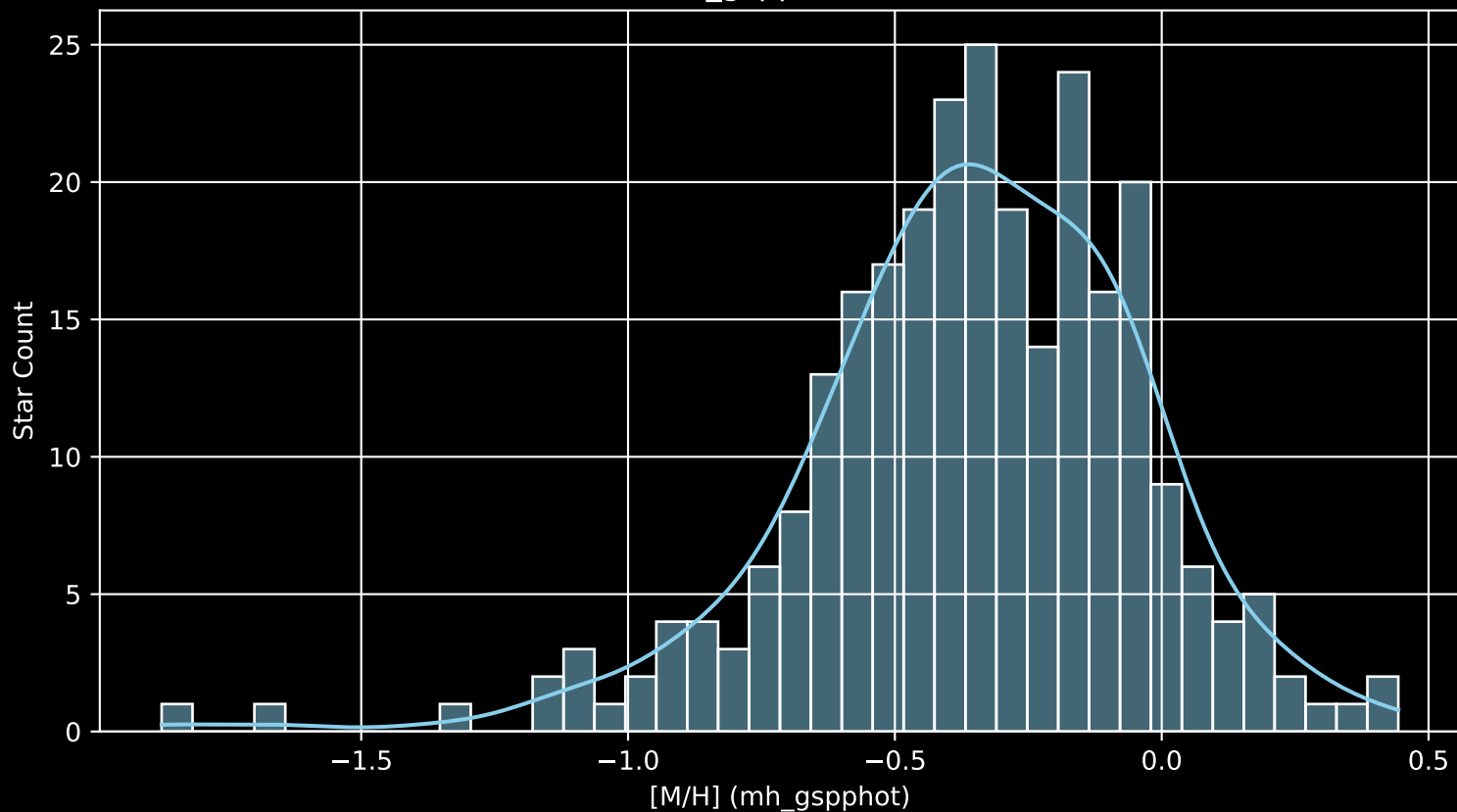
GALAH DR4 Field: [142] [M/H] (mh_gspphot) (n= 272)
