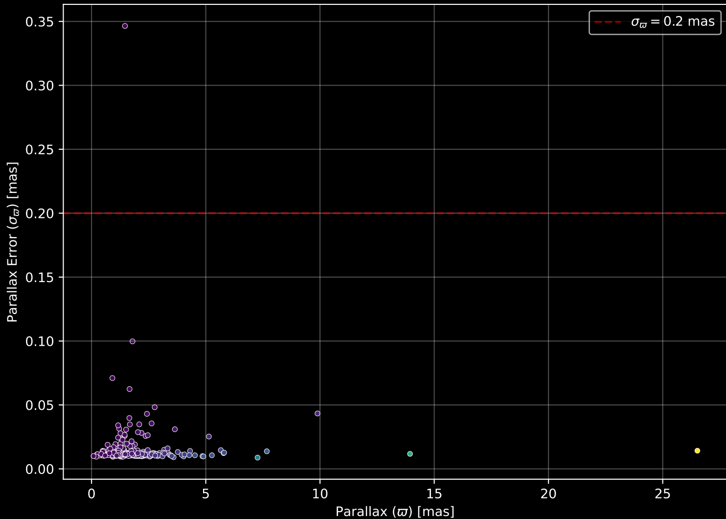
GALAH DR4 Field: [142] Parallax Quality (n= 272)
